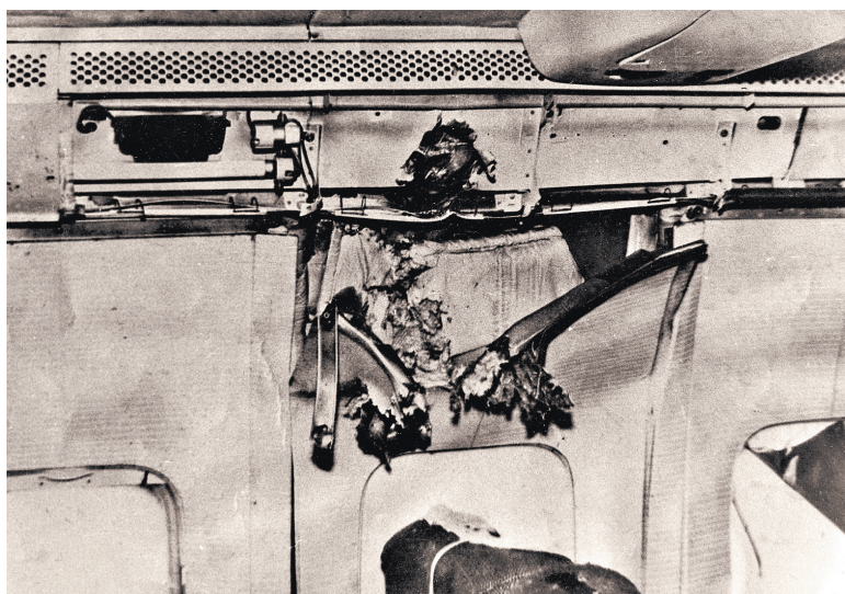
Боевая часть ракеты Р-60 стержневого типа: поражающие элементы из сплава циркония и молибдена. Сотня стержней пробили обшивку (вид из салона).
