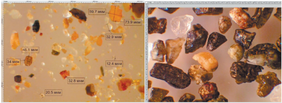
Сравнительные микроскопические изображения образца 1 (частицы силикатного песка, слева) и образца 2 (частицы магнетитового песка, справа).
